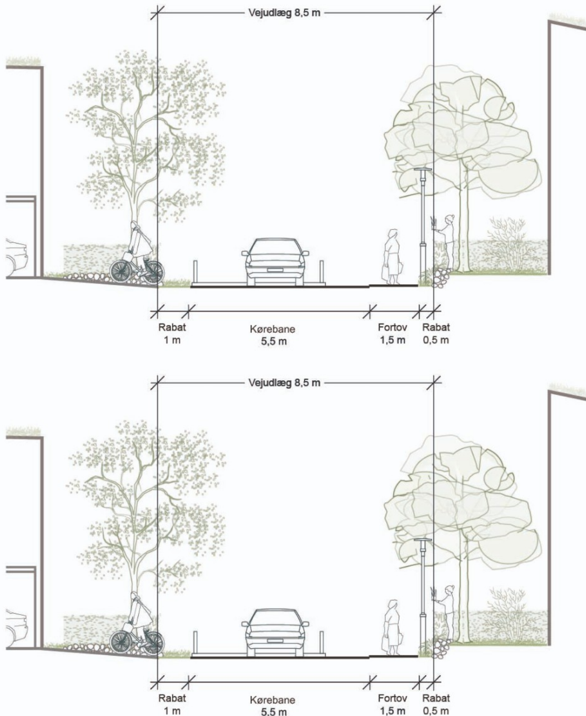
Principsnit af vej E-F
