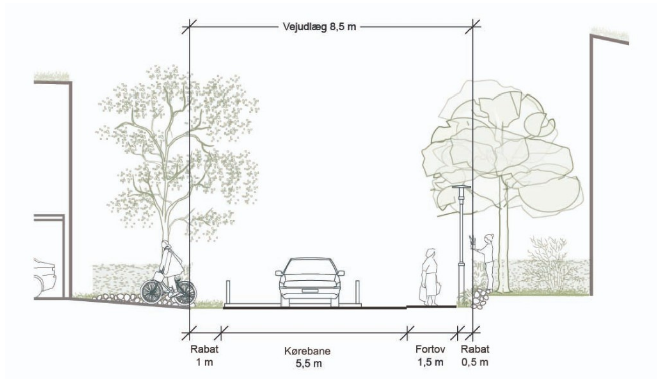
Principsnit for vejudlæg på 8,5 m.
