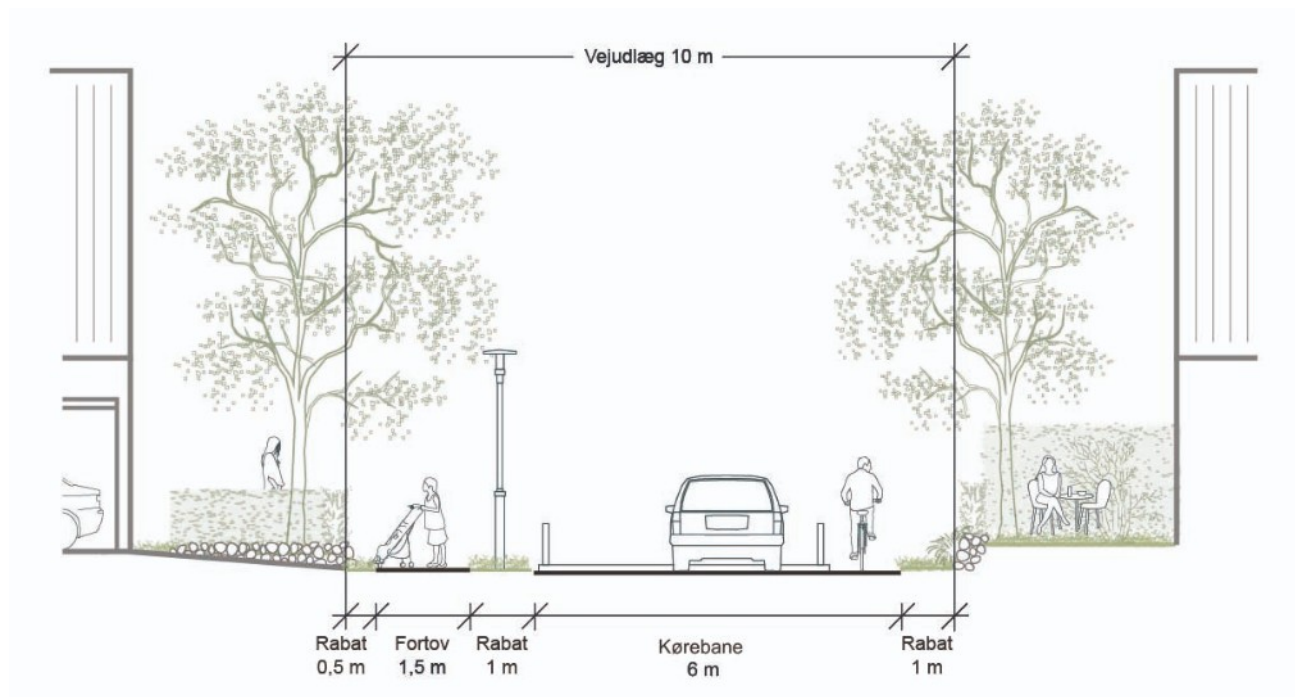
Principssnit for vejudlæg på 10 m.
