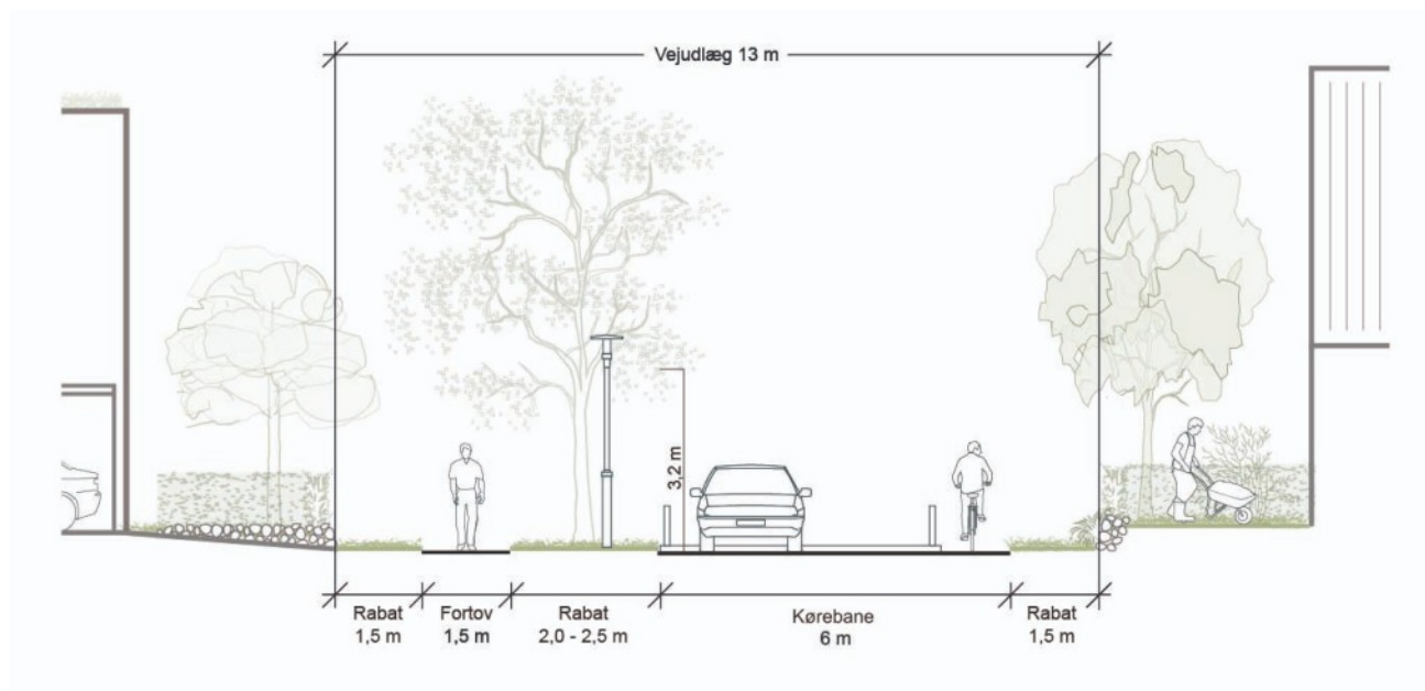
Principssnit for vejudlæg på 13 m.
