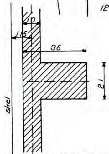
Detail „A“ 1:100 af fjv. kanal og lyre
